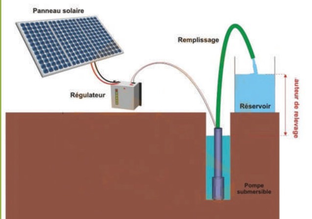
Pompe submersible - schéma de raccordement installation solaire
